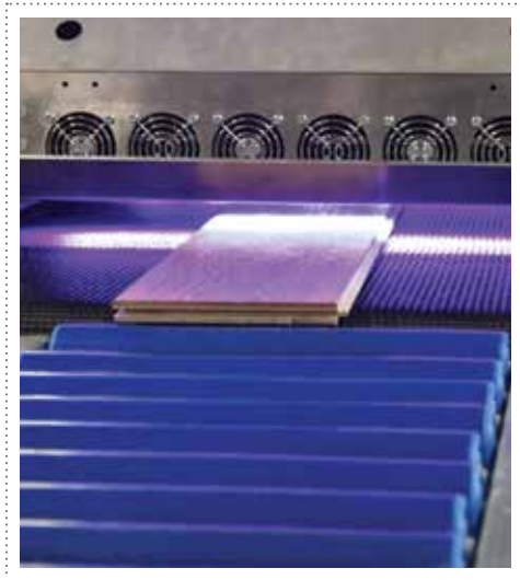
LED-CURING INDUSTRY UNIT GEÏNSTALLEERD OP DE RUBIO® MONOCOATER
